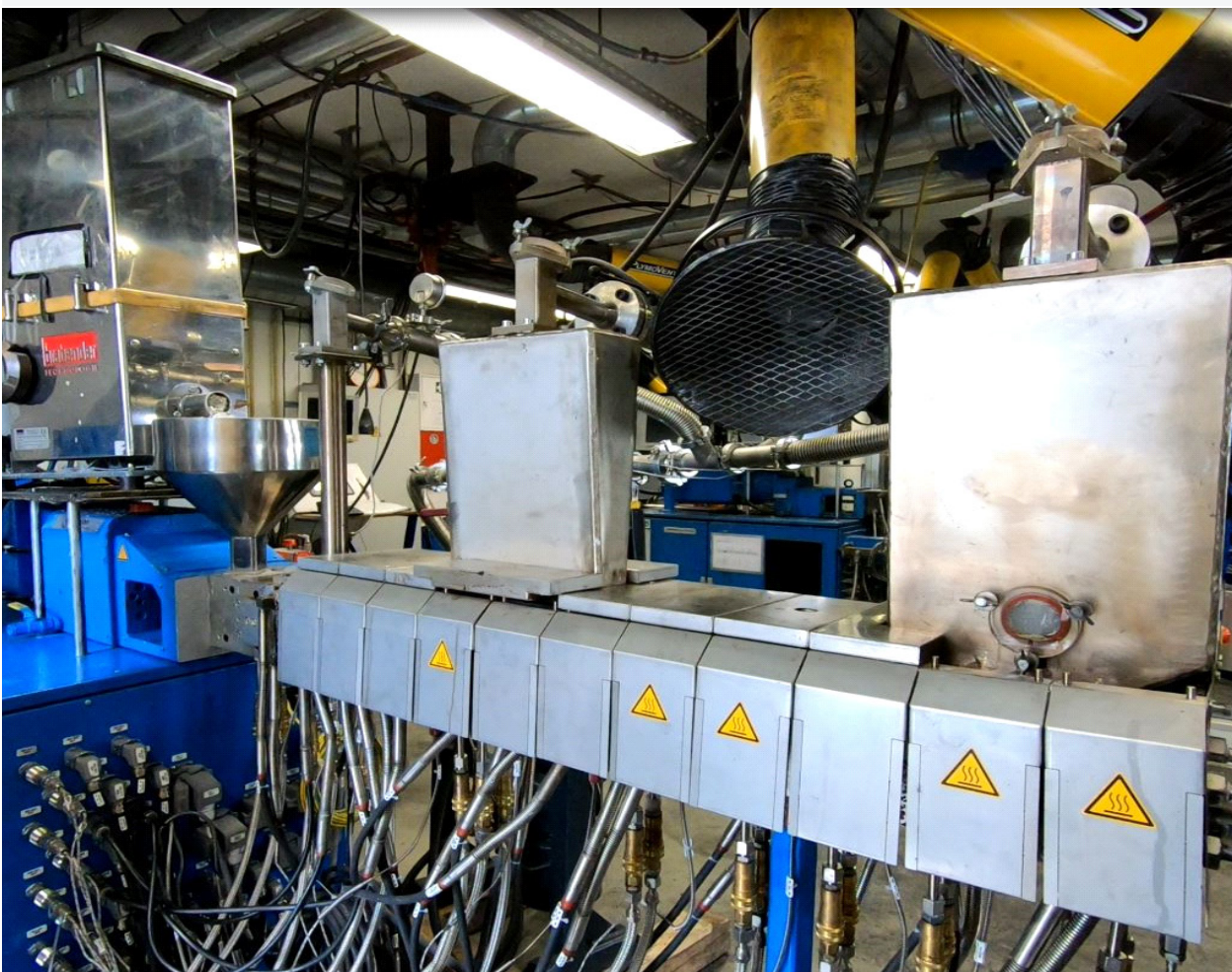
Doppelschneckenextruder zur Depolymerisation von PS-Flakes am IKV
